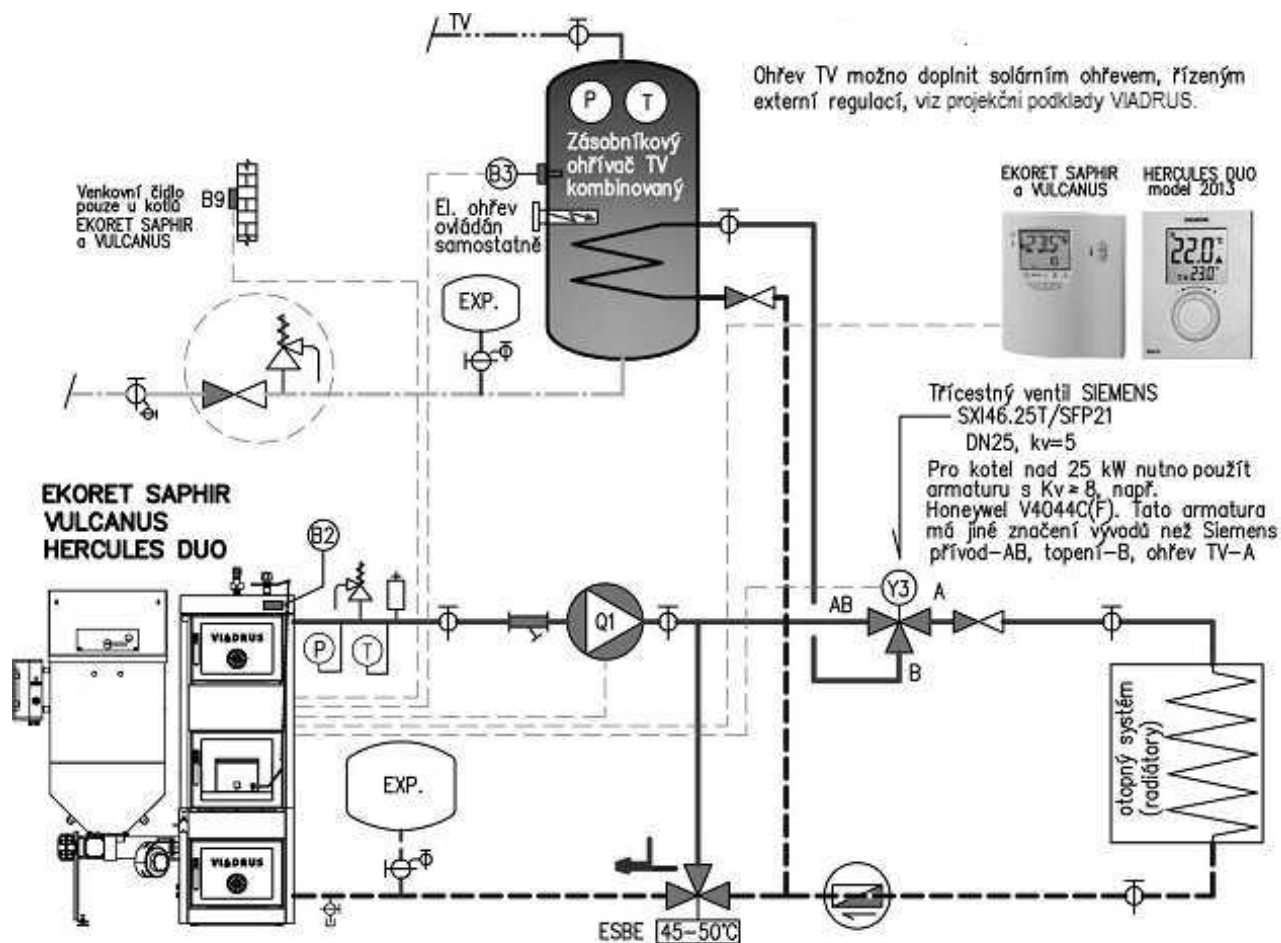
Obr. č. 6 Hydraulické schéma s přřpravou TV – řerpadlovnř topnř okruh
