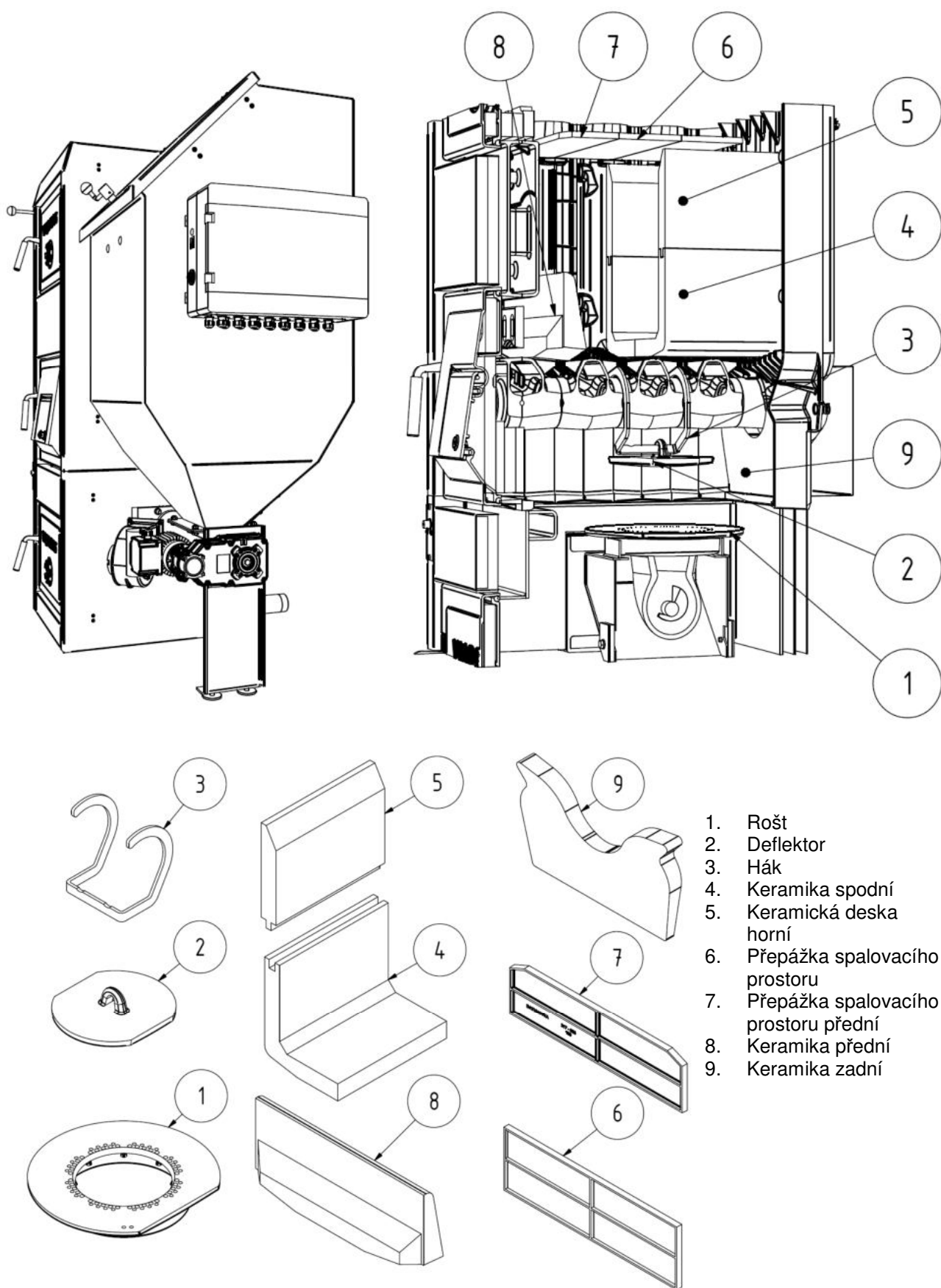
Obr. č. 11 Umístění komponent a keramik uvnitř kotle
