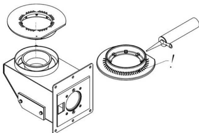
Obr. č. 17 Přestavba kotle z pravého na levé provedení – demontáž hořáku a záslepovací přírubby
