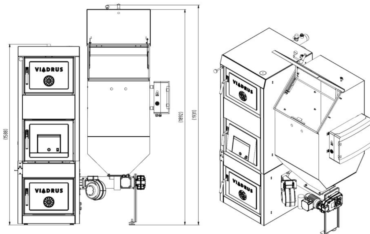
Obr. č. 5 Kotel VULCANUS (právé provedení s malým zásobníkem) s otevřeným zásobníkem paliva
