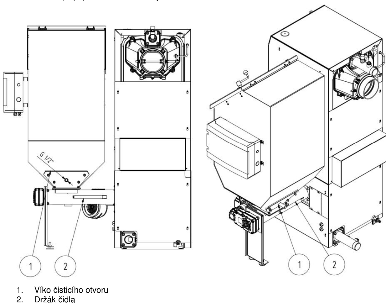
Obr. č. 15 Montáž havarijního hasicího zařízení
