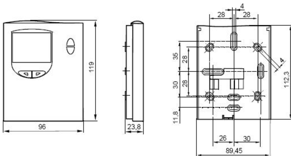
Obr. č. 25 Připojovací rozměry přístroje QAA 88 (QAX 34.3)
