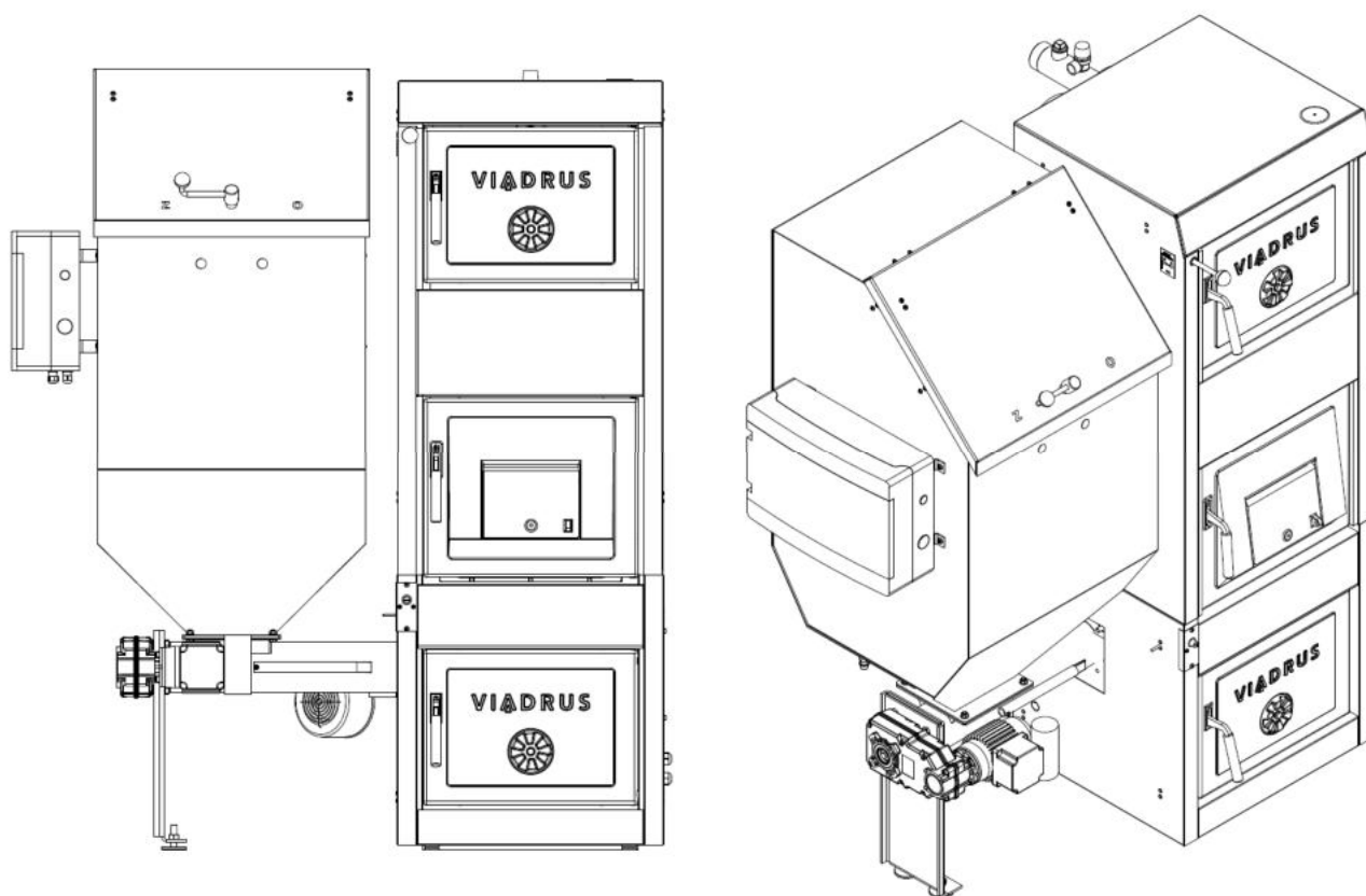
Obr. č. 18 Kotel VULCANUS (levé provedení)
