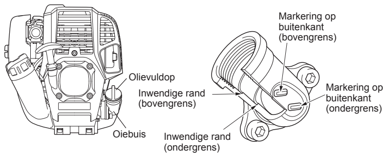
Afbeelding 2 Oliebuis
