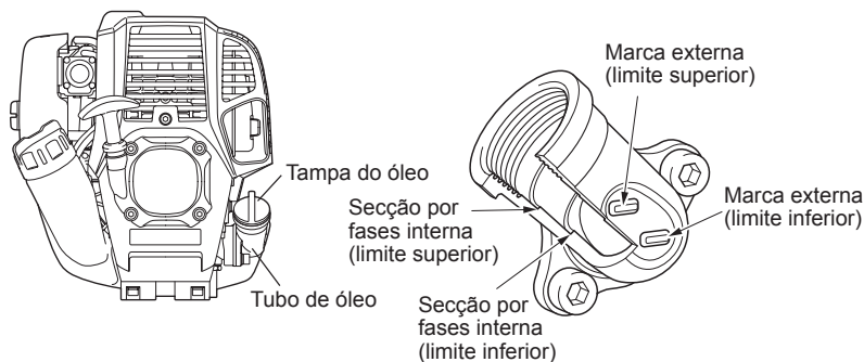
Fig. 2 Tubo de óleo
