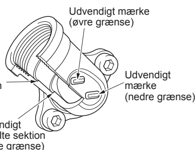
Fig. 2 Olierør
