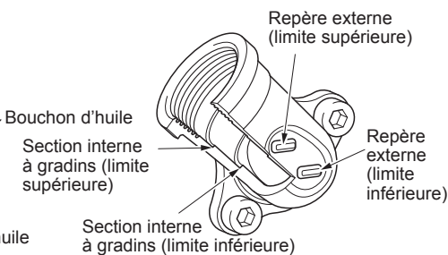
Illustration 2 Tuyau d'huile
