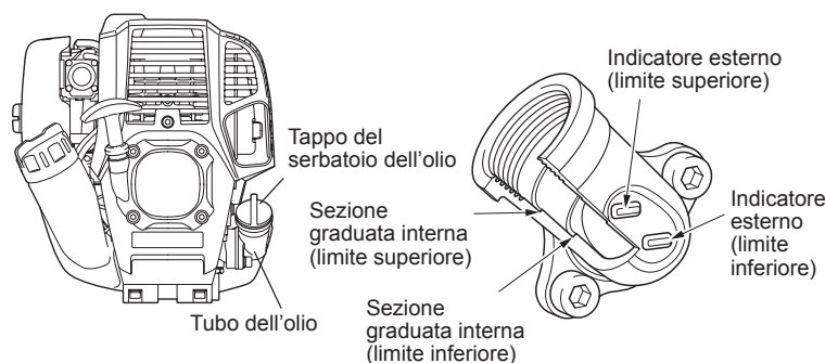
Fig. 2 Tubo dell'olio
