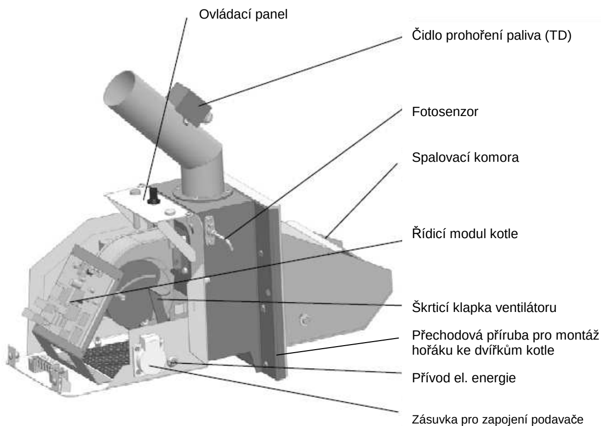
Obr. č. 6 Základní části hořáku kotle VIADRUS HERCULES Green Eco Therm XS
