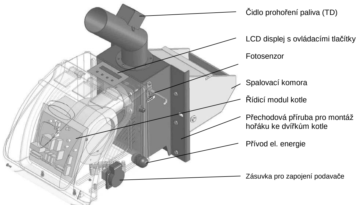
Obr. č. 5 Základní části hořáku kotle VIADRUS HERCULES Green Eco Therm XJ
