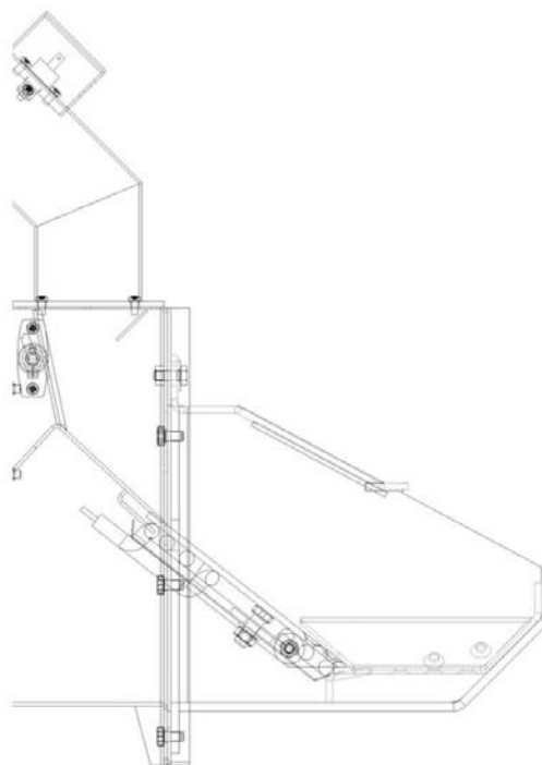
Obr. č. 24 Konečné umístění roštu
