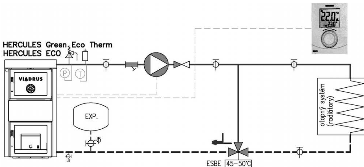
Obr. č. 19 Hydraulické schéma kotle VIADRUS HERCULES Green Eco Therm
