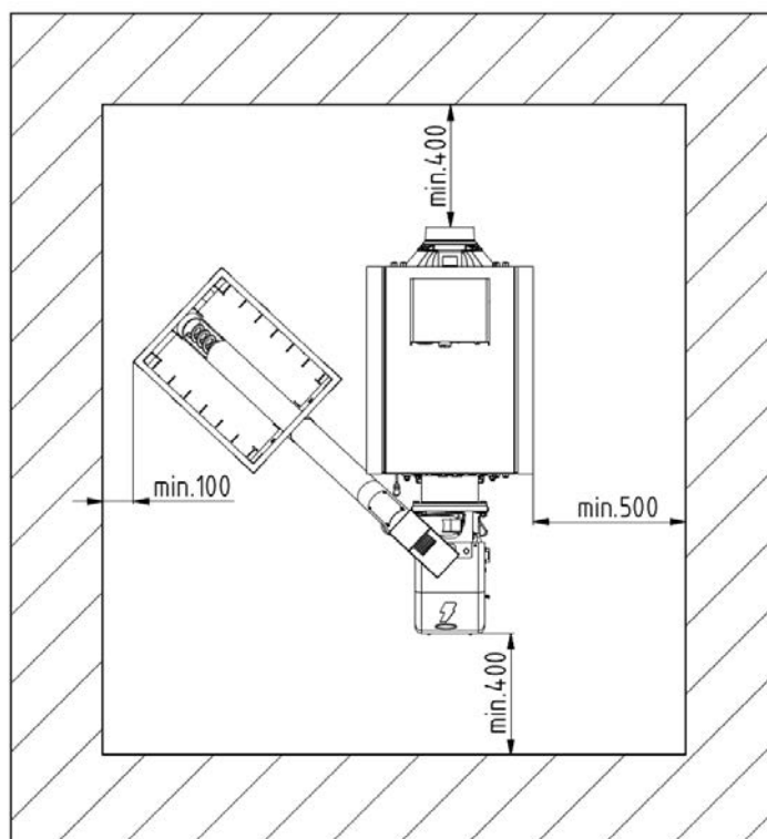
Obr. č. 9 Umístění kotlů v kotelně
